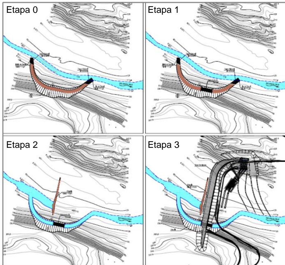
Figura 3-1. Etapas del desvío de la Presa Kirchner (UTE Optimizado)
