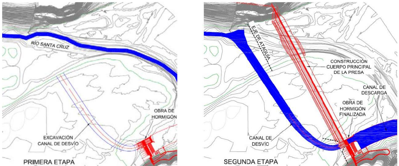
Figura 3-2. Etapas del desvío para Cepernic.
